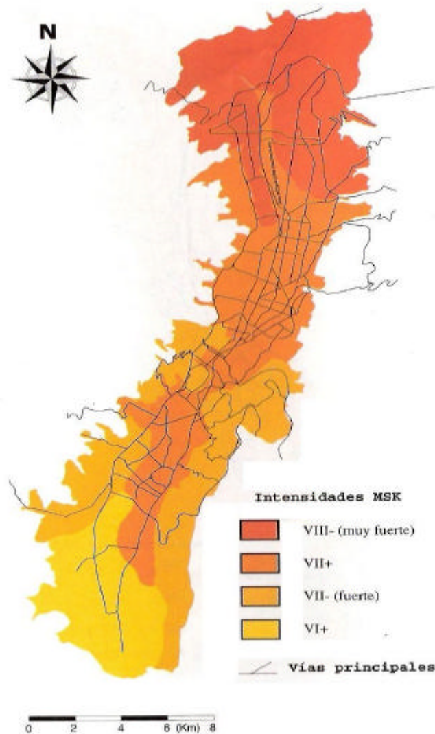
FIGURA 6. INTENSIDADES EN QUITO POR EL SISMO LOCAL (SL)
