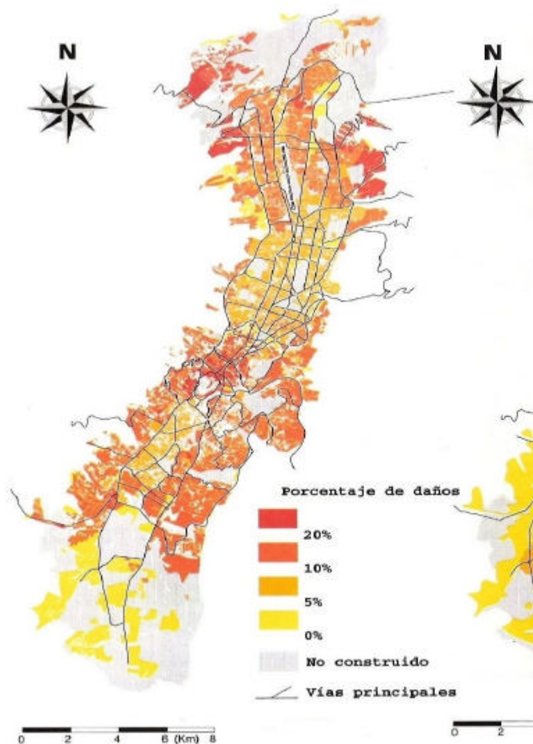
FIGURA 8. ESTIMACIÓN DE DAÑOS A LAS CONSTRUCCIONES PROVOCADOS POR EL SISMO LOCAL
