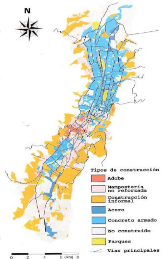
FIGURA 7. DISTRIBUCIÓN DE LOS TIPOS DE CONSTRUCCIÓN
