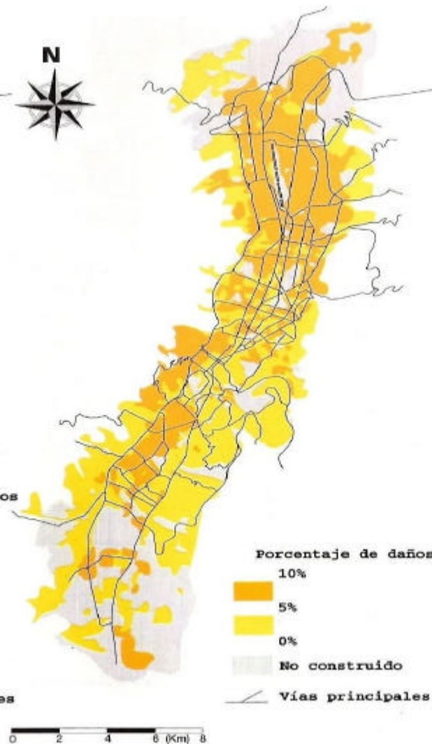
FIGURA 9. DAÑOS A LA CONSTRUCCIÓN PROVOCADOS POR EL SISMO DE 1987
