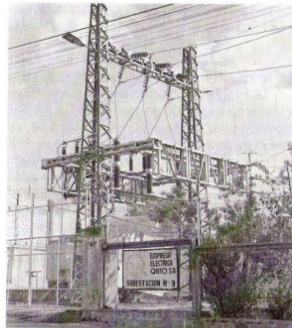
SUBESTACION ELÉCTRICA.
