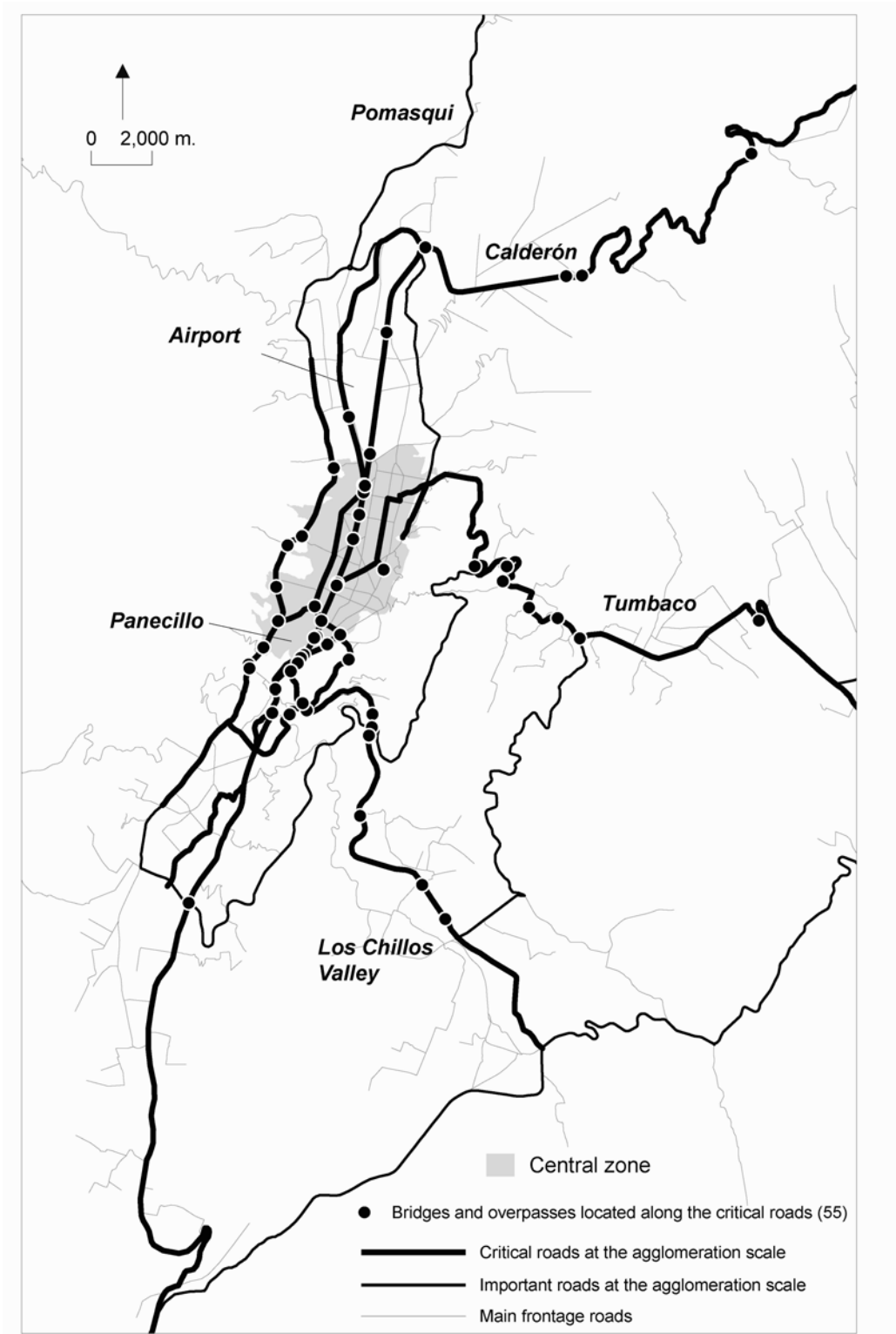
Carte 1 – Ponts et passages surélevés situés le long des axes enjeux. Map 1 – Bridges and overpasses located along the critical roads.
