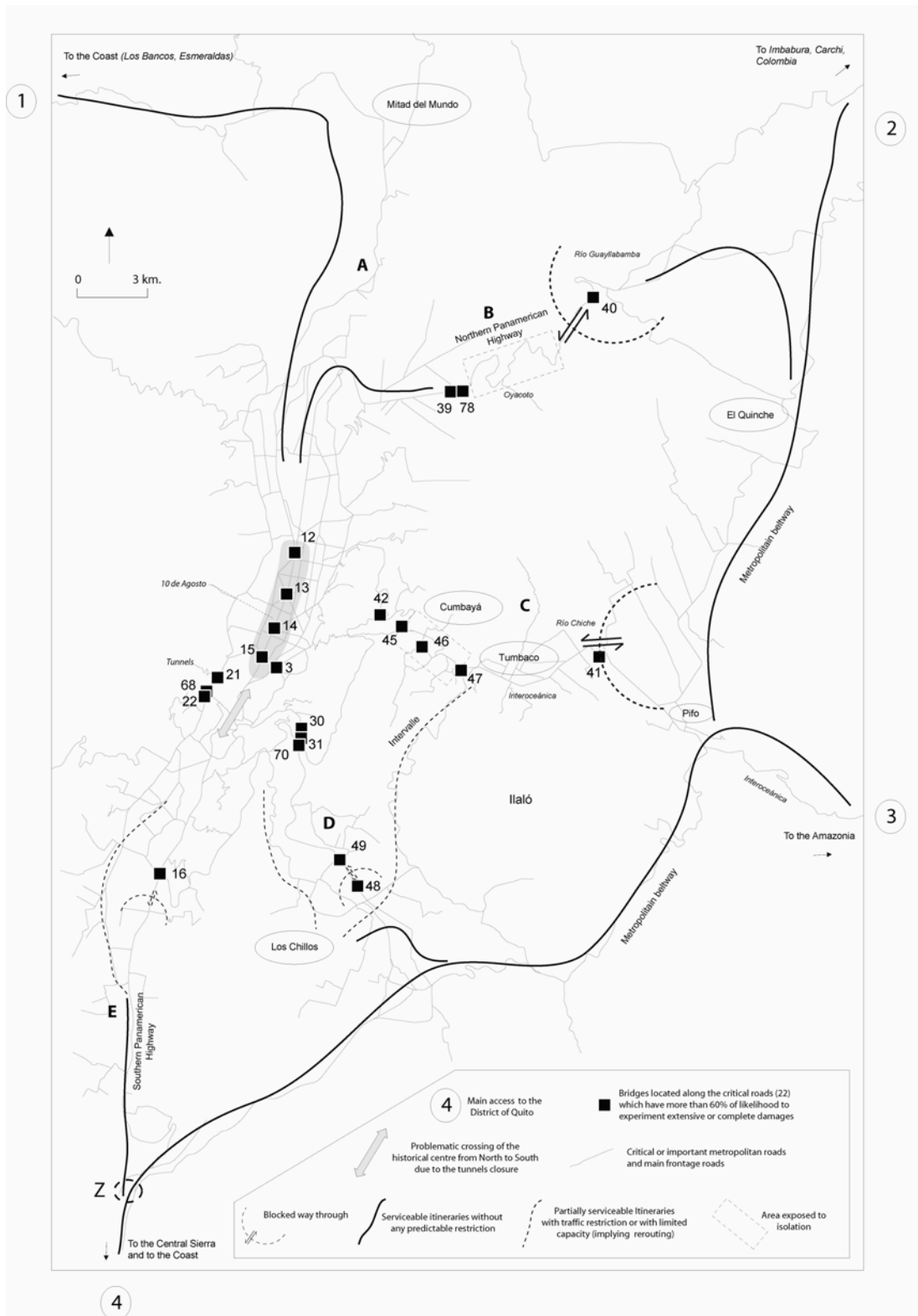
Carte 3 – Scénario des perturbations possibles de la mobilité provoquées par la fermeture des axes en jeu compte tenu de l'effondrement des ponts en cas de séisme très sévère (PGA = 0,40g) dans le district de Quito. Map 3 – Scenario of possible disruptions of mobility derived from the closure of the critical roads resulting from the collapse of bridges and overpasses in case of a very severe earthquake (PGA = 0.40g) in the Quito district.
